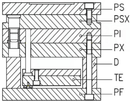
TIPO XE
