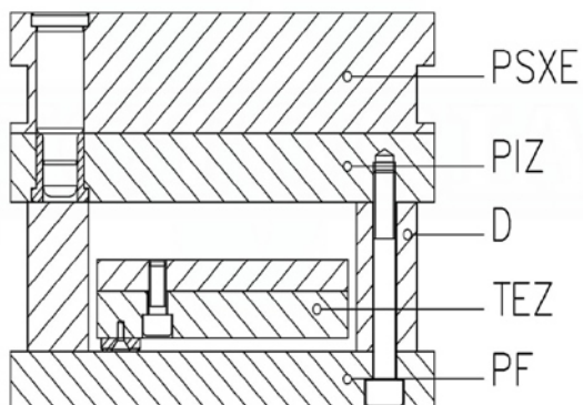
TIPO XEZ
