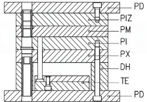
TIPO XEM
