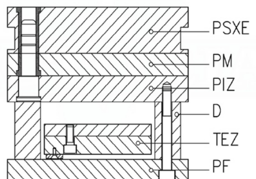
TIPO XEZM
