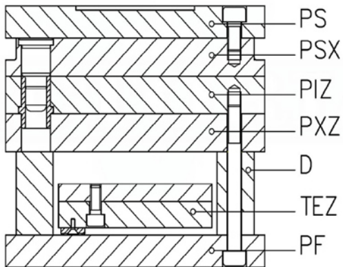
TIPO XEZ
