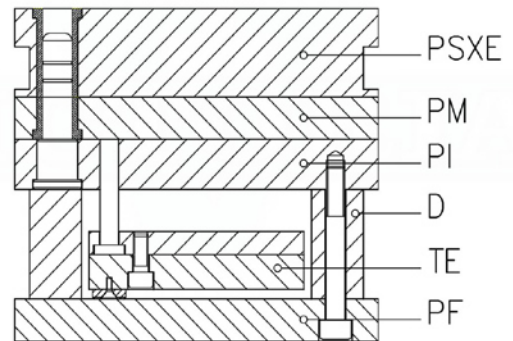
TIPO XZM
